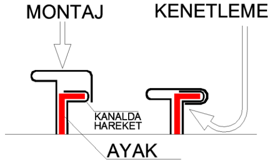
KENET BİRLEŞİM DETAYI
