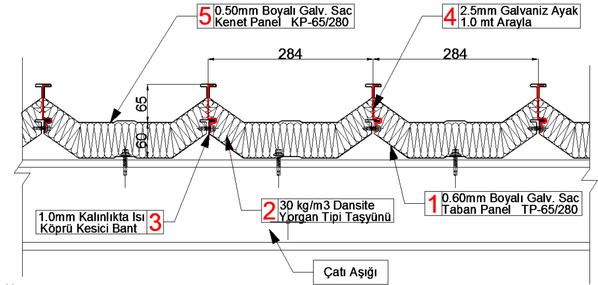
KSPS(KENTLİ SANDVİÇ PANEL SİSTEMİ) TİPİK ÇATI SİSTEM KESİTİ
